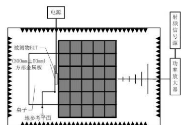
射频电磁场辐射抗扰度(80MHz 至 2.7GHz)
