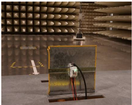
射频辐射骚扰
