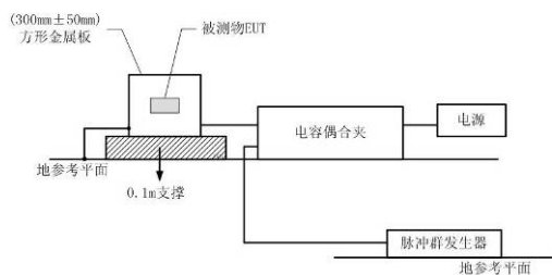
电快速瞬变 / 脉冲群抗扰度
