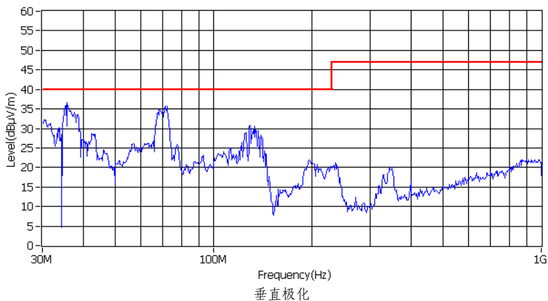
射频辐射骚扰预扫描曲线(峰值)
