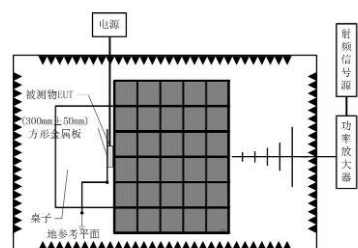
射频电磁场辐射抗扰度
