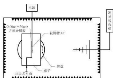
高频发射极限(30MHz 至 1000MHz)
