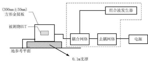
浪涌抗扰度
