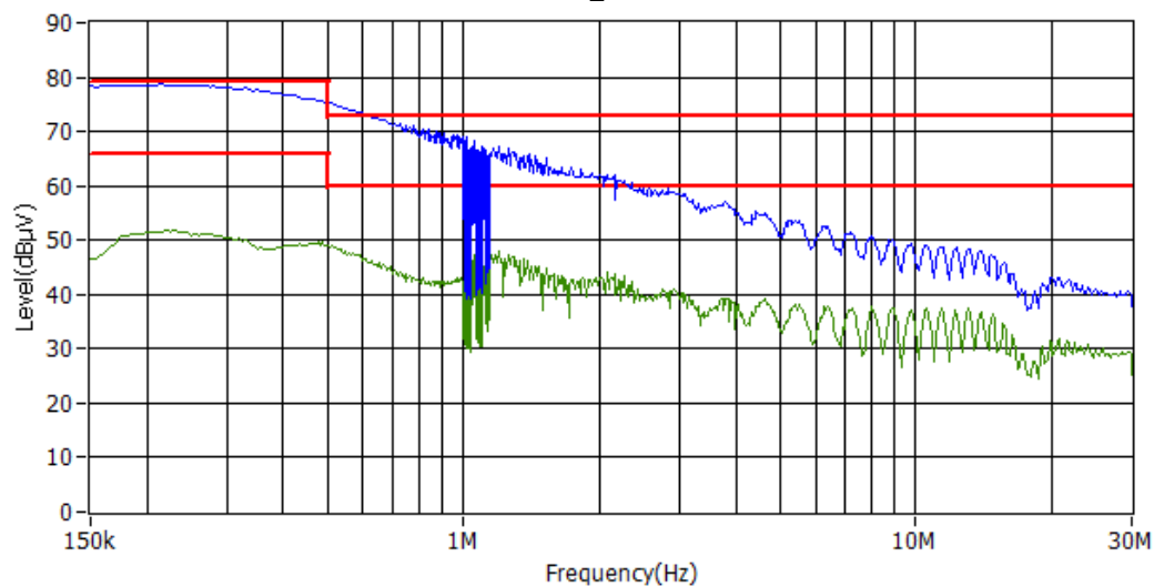
射频传导骚扰电压预扫描曲线(峰值)
