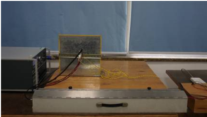
电快速瞬变 / 脉冲群
