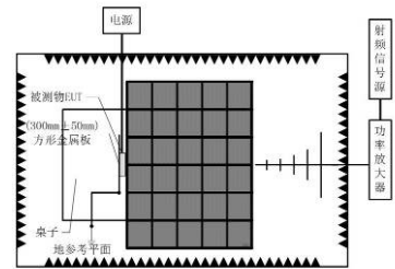
射频电磁场辐射抗扰度(80MHz 至 2.7GHz)
